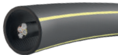
Extena Prefab Kraft. SRS kabelskyddsror med fördragen kraftkabel (4G25 AL).
